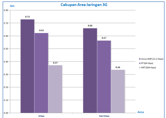
Gambar 20 Cakupan Area 3G Area Urban dan Sub-Urban
