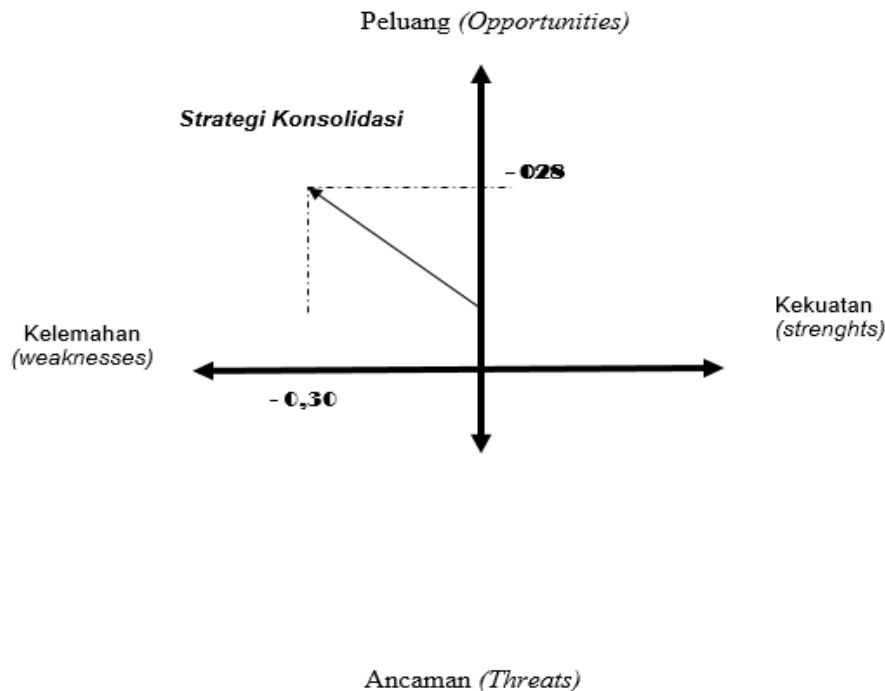
Gambar 10. Hasil analisa SWOT
