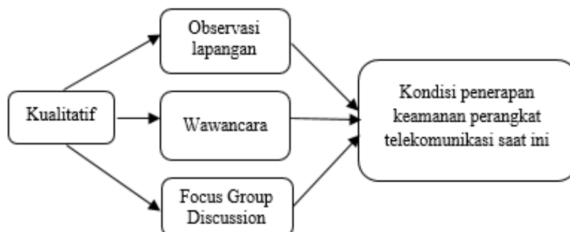
Gambar 1. Metode kualitatif
