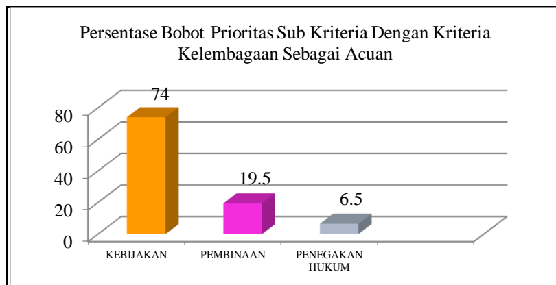
Gambar 8. Bobot sub kriteria dengan kriteria kelembagaan sebagai acuan
