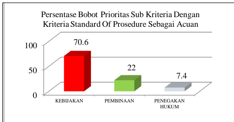
Gambar 5. Bobot sub kriteria dengan kriteria SOP sebagai acuan
