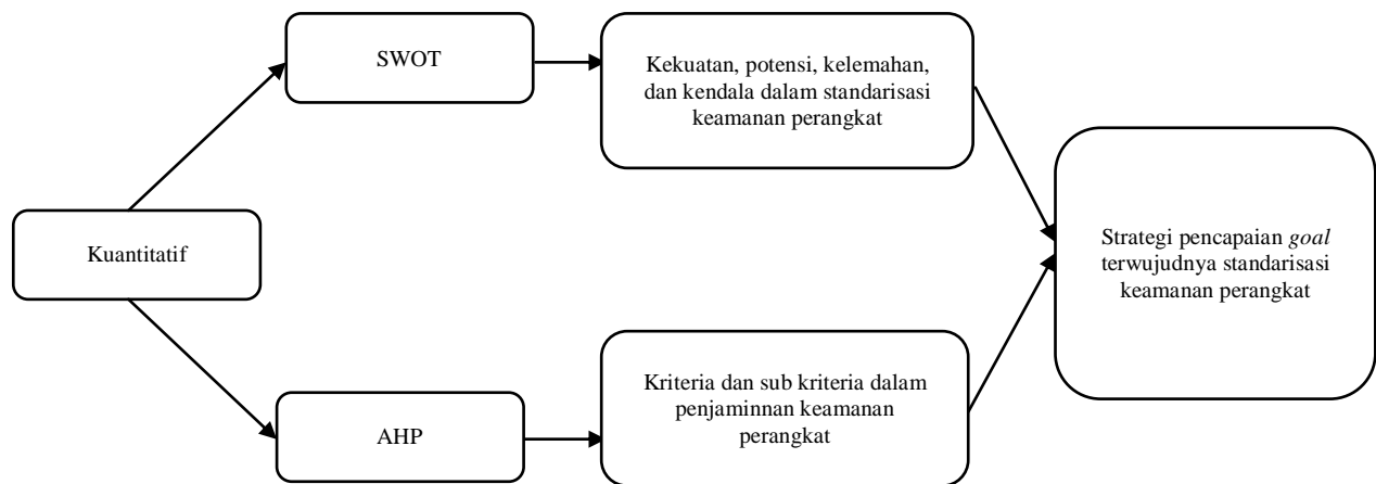
Gambar 2. Metode kuantitatif
