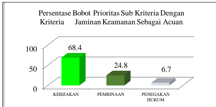
Gambar 6. Bobot sub kriteria dengan kriteria jaminan keamanan sebagai acuan
