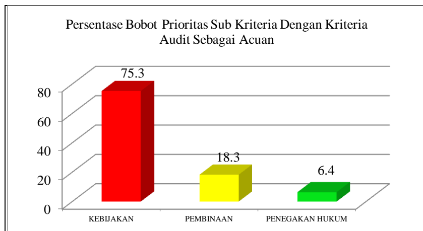
Gambar 9. Bobot sub kriteria dengan kriteria audit sebagai acuan
